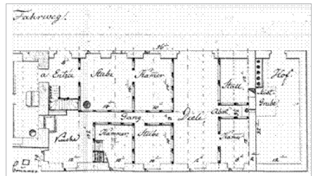
Grundriss der Lehrerwohnung mit anschließendem Stallteil.
